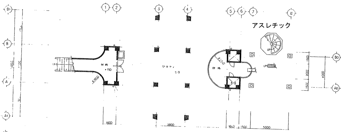
1階平面図 S=1/100
