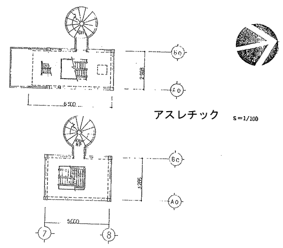
アスレチック S=1/100
