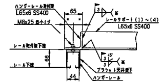
ハンガーレール取付詳細
