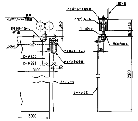
カーテン(1) 用レール取付詳細
