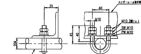
カーテン(2) 用レール取付Uボルト 詳細
