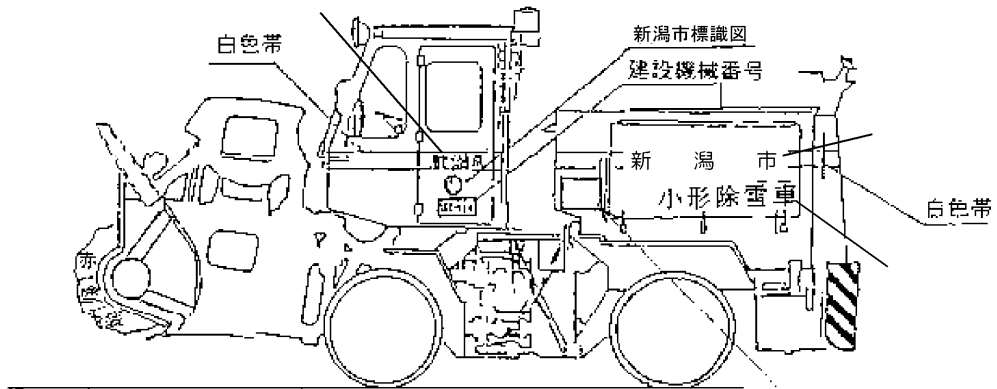
図1 除雪機械表示箇所図
