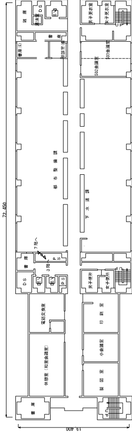
4階 平面図
