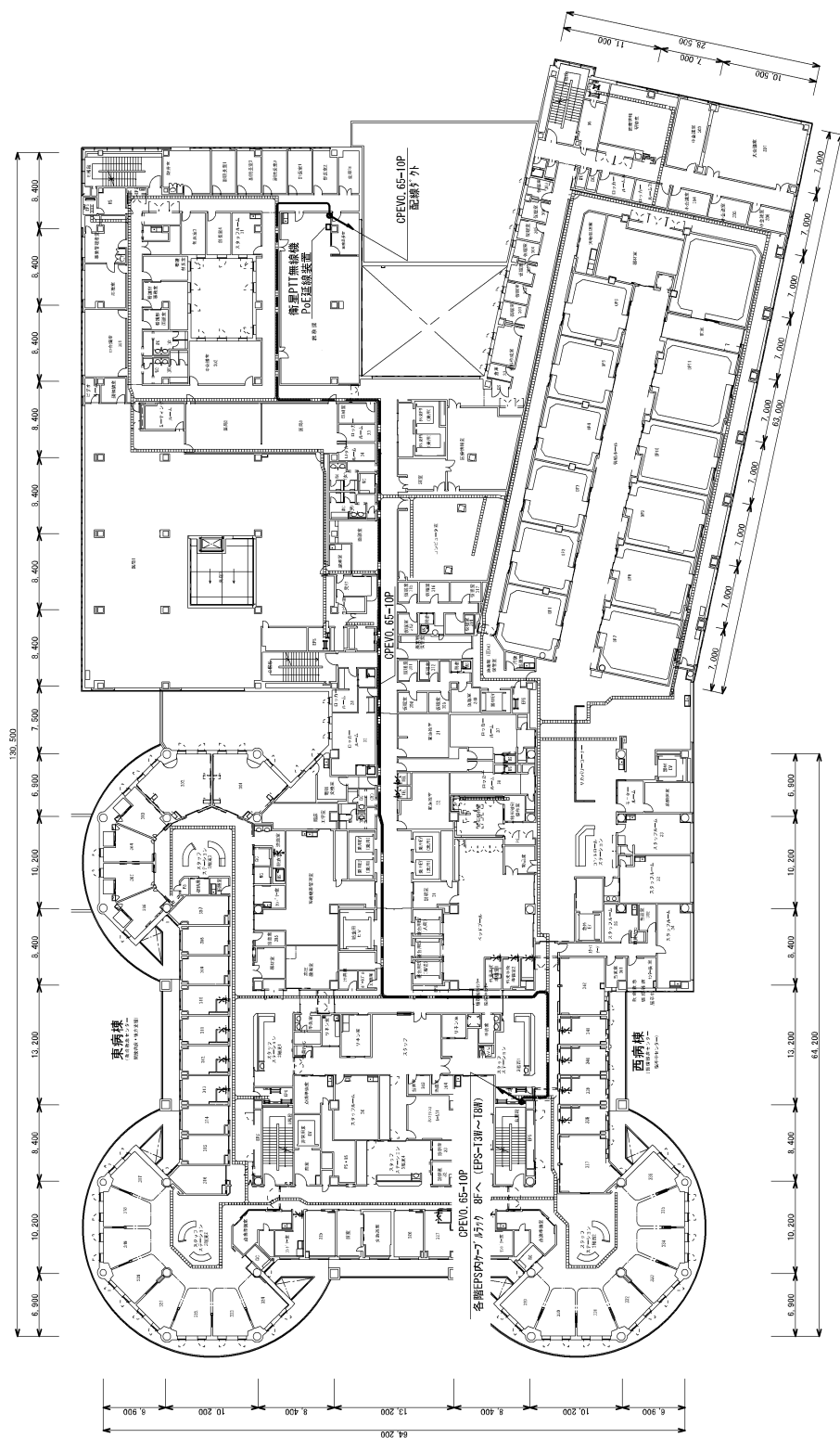
3 F 平面図
