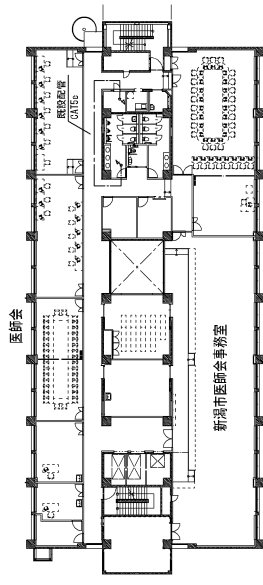
5階 平面図
