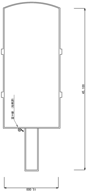
PH 平面図
