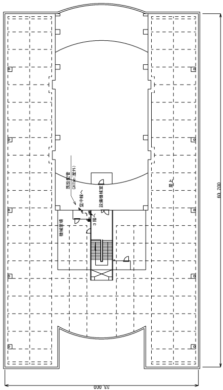
屋上 平面図
