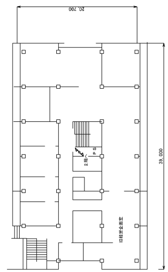
3階 平面図
