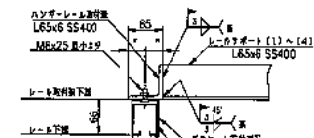
ハンガーレール取付詳細
