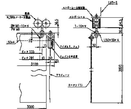
カーテン(1)用レール取付詳細
