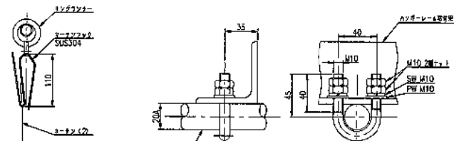
カーテン(2)取付部 カーテンフック詳細
