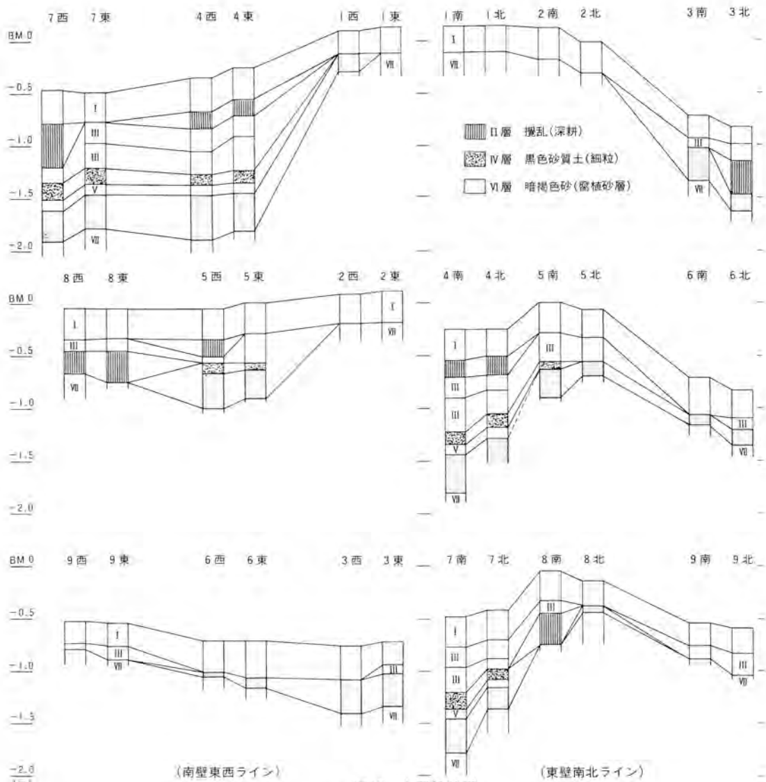
図26 土層柱状図
