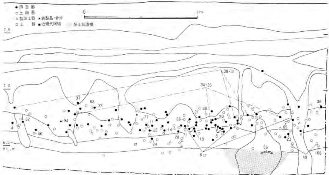
図5 第6トレンチ遺物垂直分布(西壁土層図に遺物・焼土状遺構を投影)
