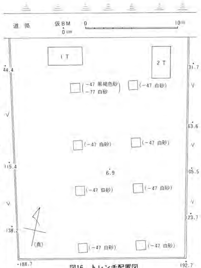
図16 トレンチ配置図
