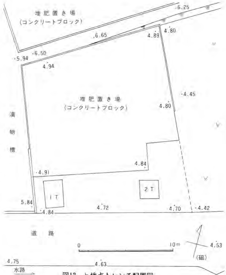
図13 b地点トレンチ配置図
