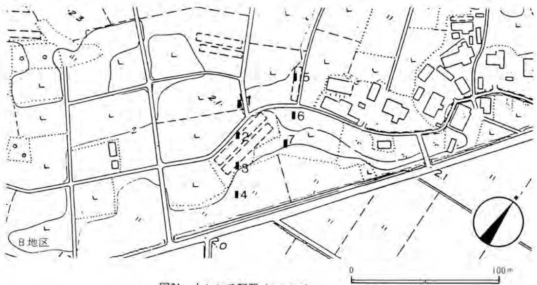
図21 トレンチ配置 (1/2,500)
