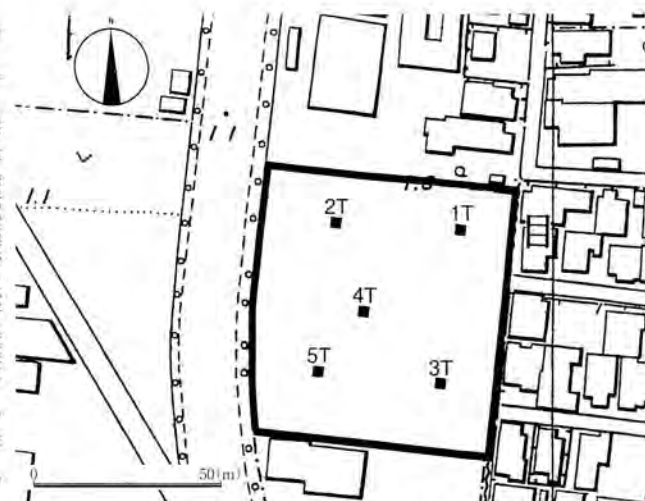
図32 試掘坑配置図 (S=1/2,000)
