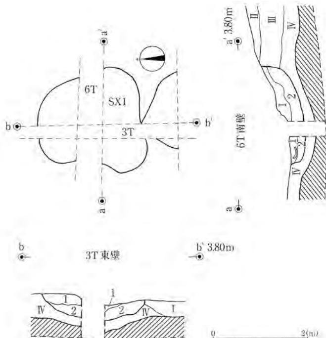
図43 SX1検出状況 (S=1/40)
