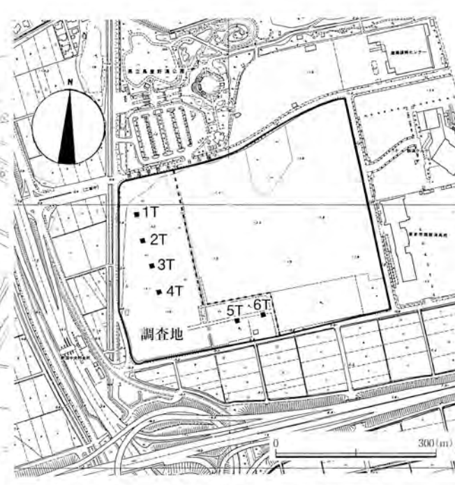
図17 試掘坑位置図（S=1/10,000）
