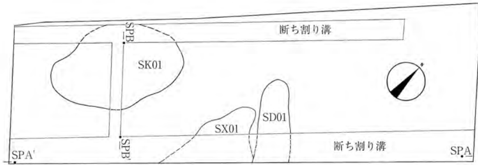
図6 1T遺構平面図 (S=1/40)
