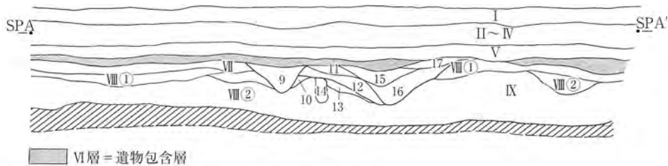
図7 SD01及びSX01にかかる土層堆積状況図 (S=1/40)
