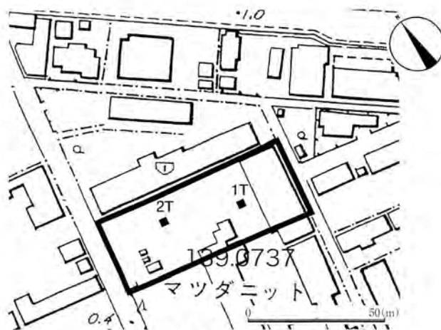
図36 試掘坑配置図 (S=1/2,000)
