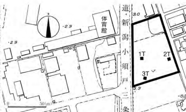
図34 試掘坑配置図 (S=1/3,000)
