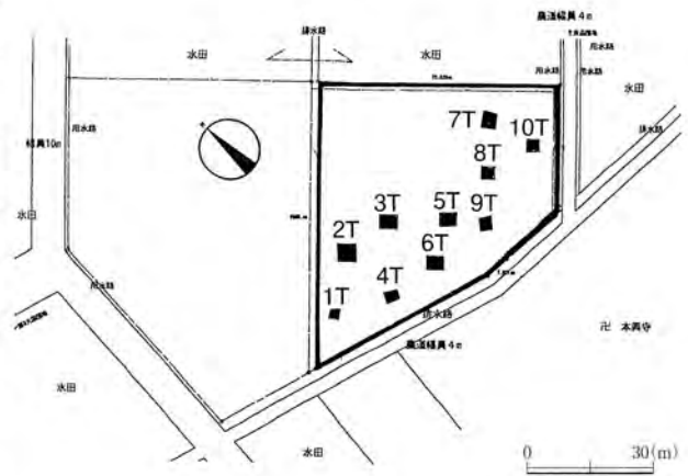
図30 試掘坑位置図 (S=1/1,500)
