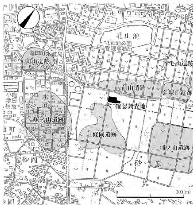
図12 調査地位置図 (S=1/10,000)
