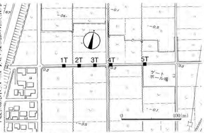
図26 試掘坑位置図 (S=1/4,000)
