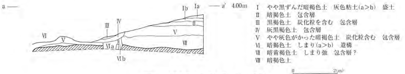
図41 1T土層堆積状況図 (S=1/50)
