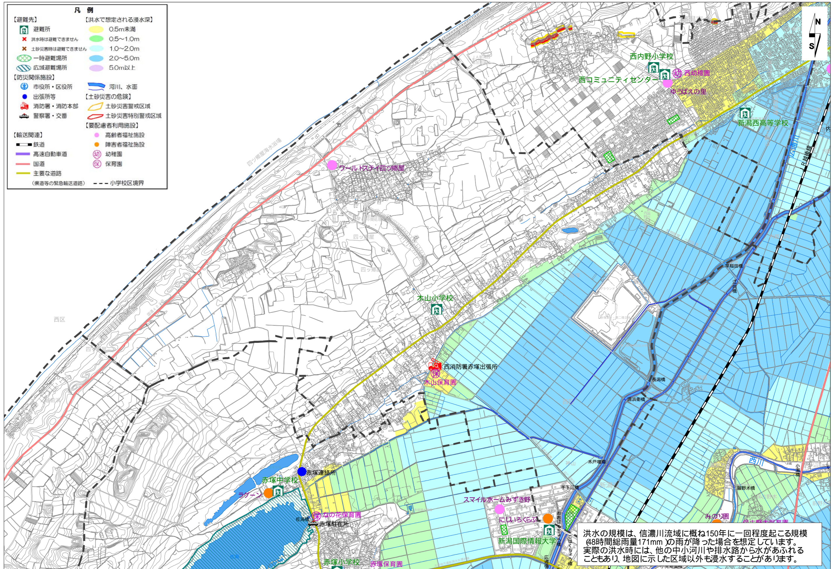
様式6-1 風水害（洪水・土砂災害）対策地図（大河津分水路）
