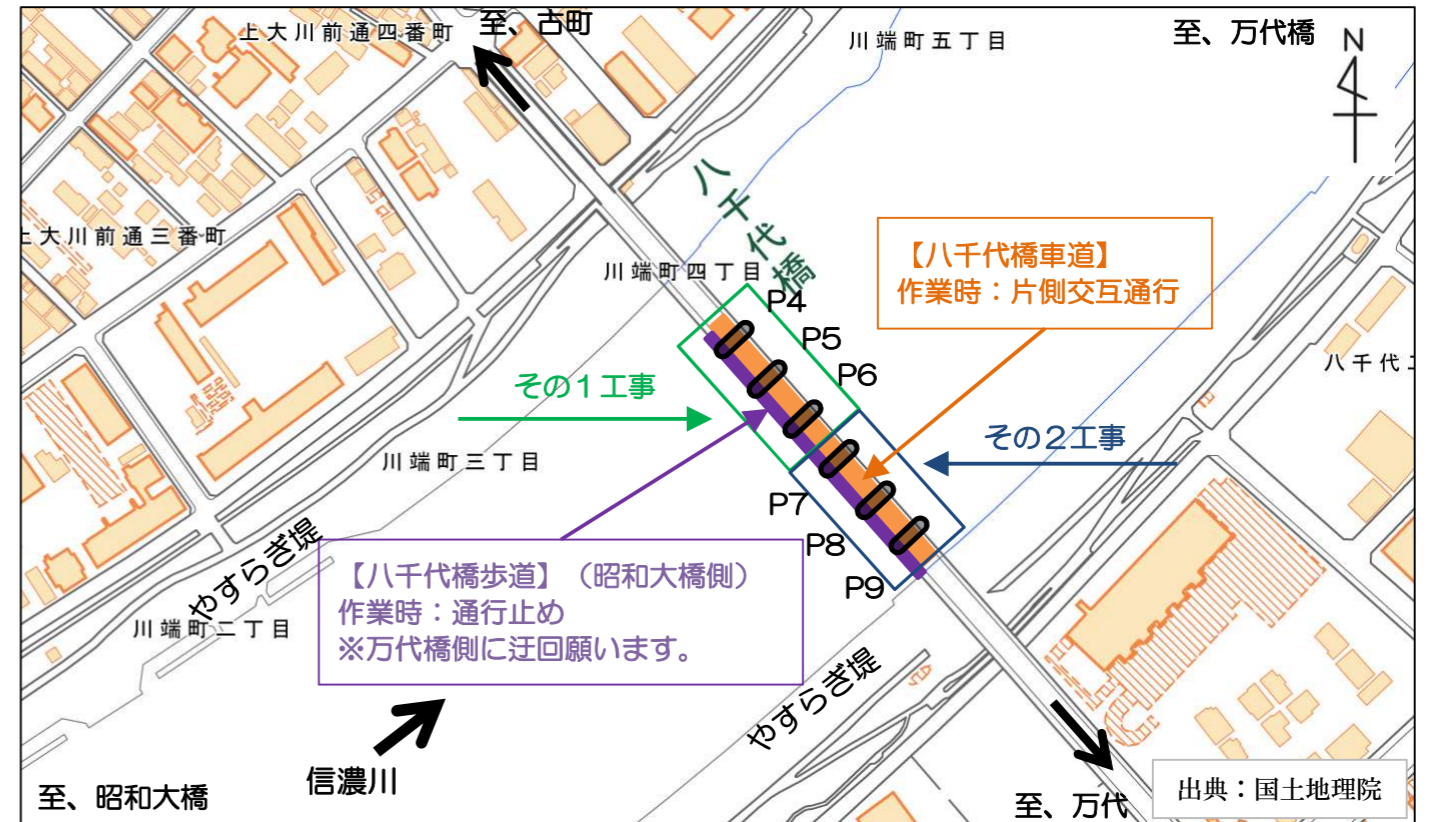
補修箇所（橋脚）
