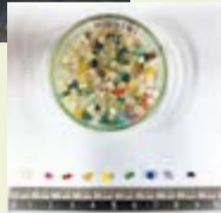
▶新潟の海岸で確認されたマイクロプラスチック
