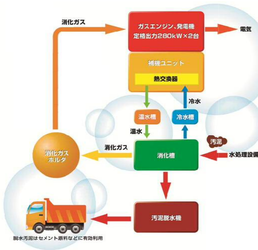
【消化ガス発電の概要図】
