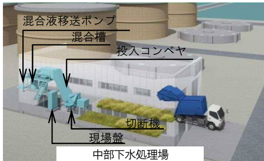
中部下水処理場
