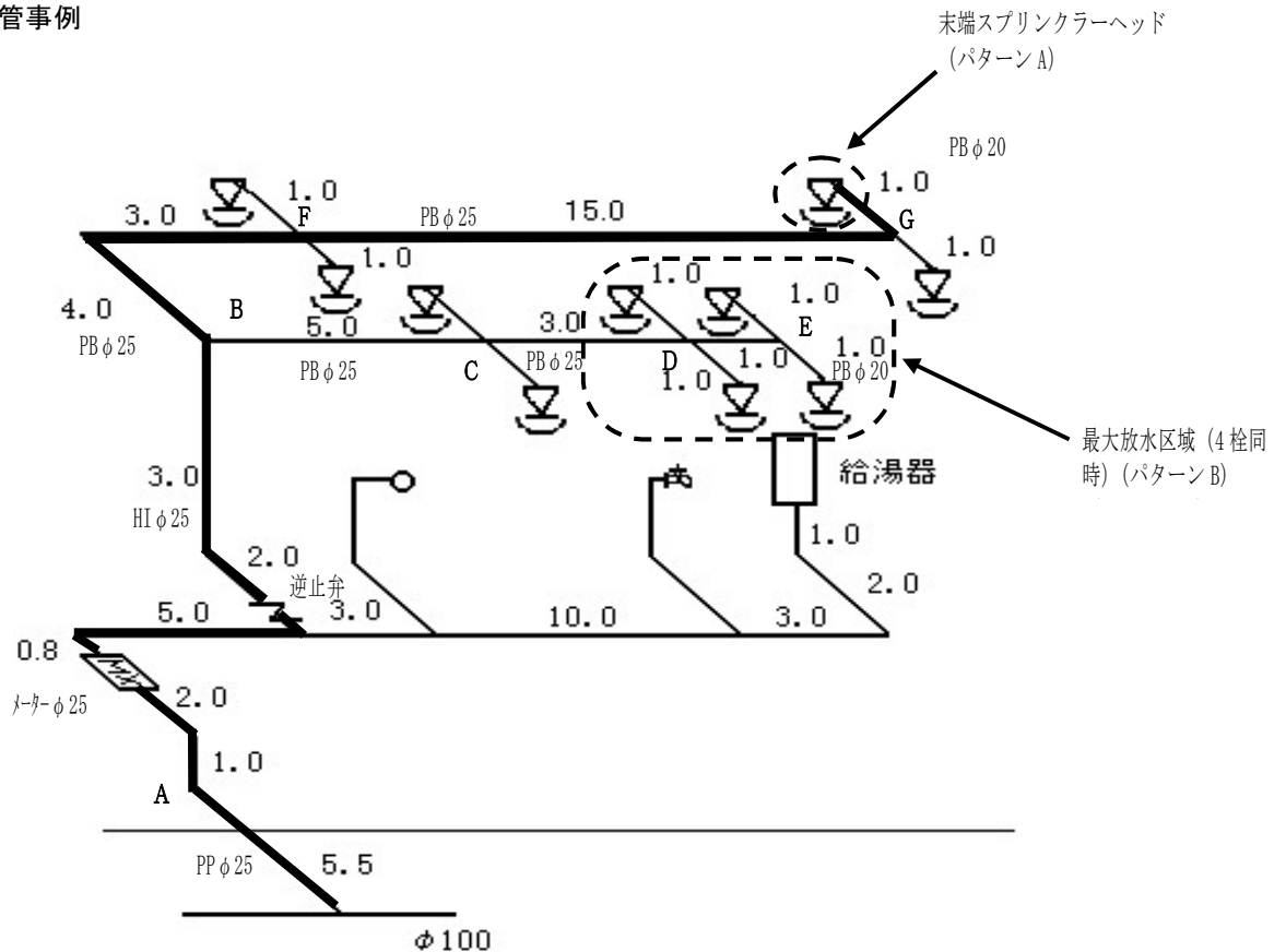
図-1 配管事例
