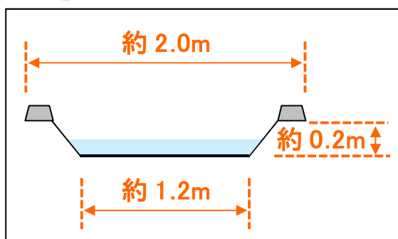
【「ど」の基本寸法】
