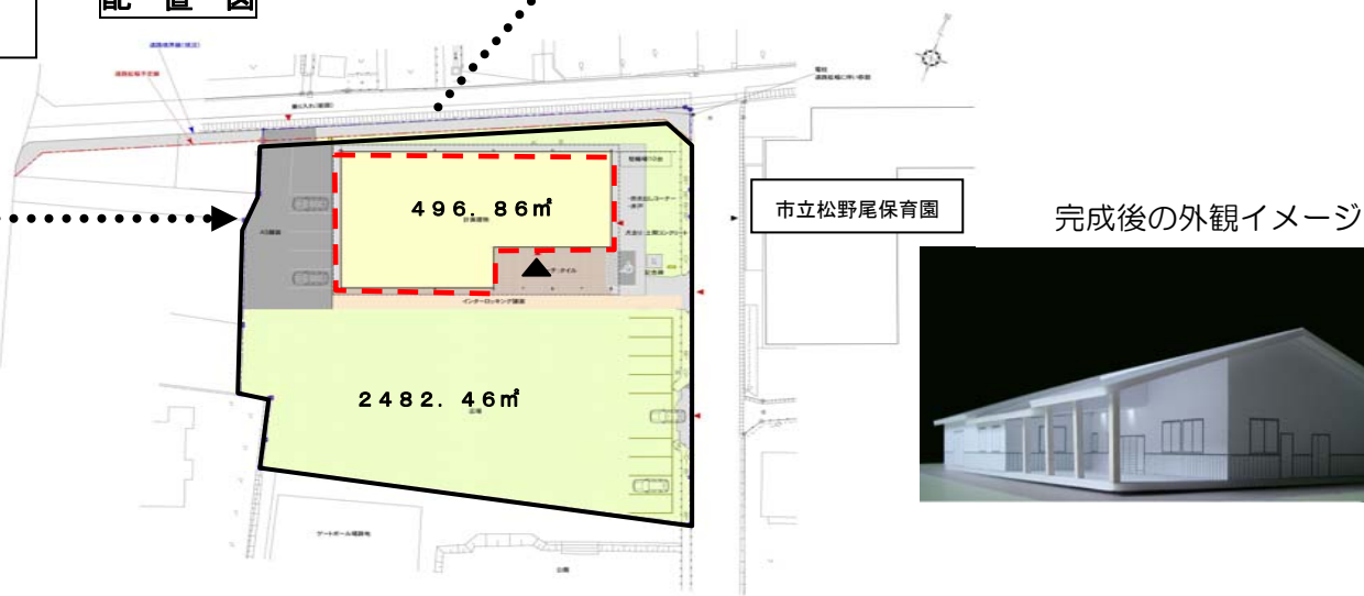
配置図
