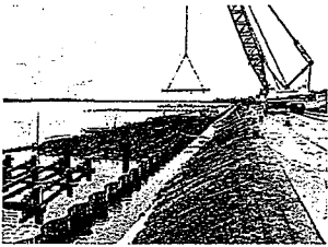
9月粗礫沈設
