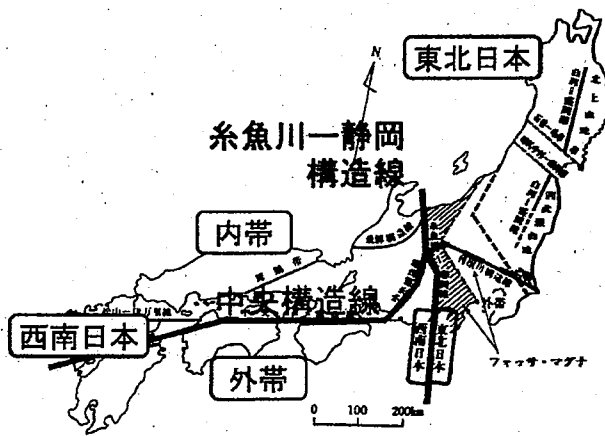
図 2.14 日本の地質構造区分
