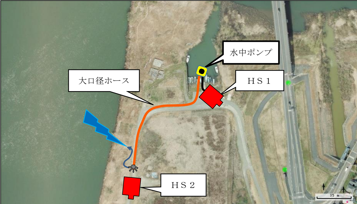
【詳細図】
